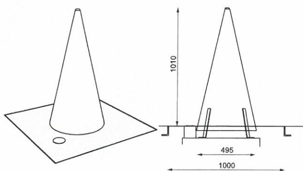
HD310: nerezový kužel, kotvení do trativodového čtverce
