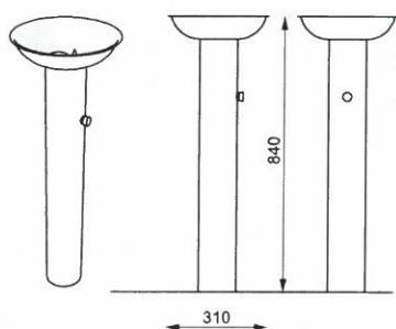
HD210: nerezový sloupek s miskou, kotvení pod dlažbu
