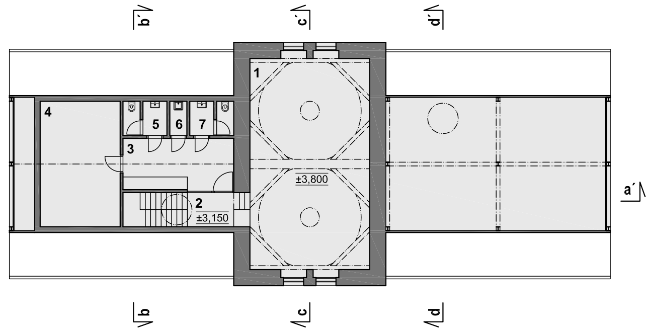
1 - univerzální kulturní prostor (galerie/klubovna), 2 - schodiště, 3 - kuchyně, 4 - sklad galerie, 5 - WC muži, 6 - úklid, 7 - WC ženy
