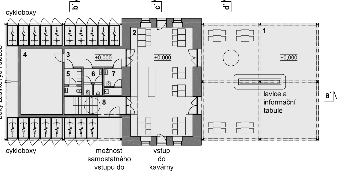
1 - přístřešek čekárny autobusových zastávek, 2 - kavárna, 3 - chodba, 4 - sklad kavárny, 5 - zázemí zaměstnanců, 6 - WC muži, 7 - WC ženy, 8 - schodiště
