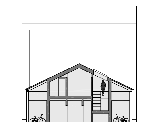
řez b-b', m 1:200
