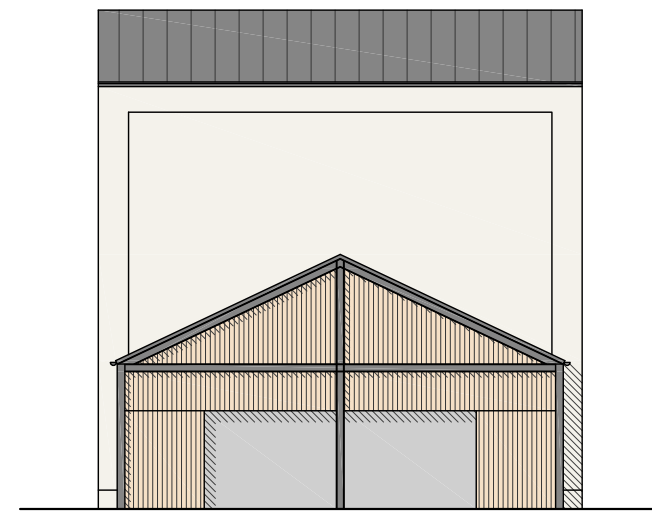
pohled jižní, m 1:200
