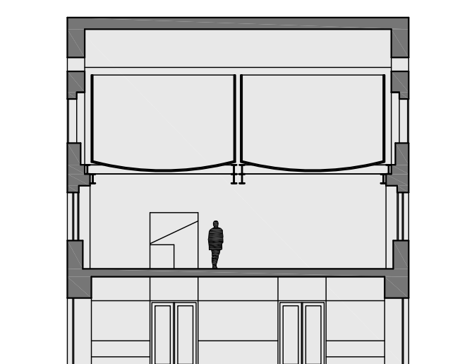
řez c-c', m 1:200
