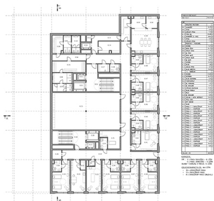
PŮDORYS 2NP M 1:200
