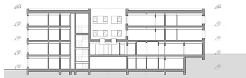
ŘEZ B-B' M 1:200
