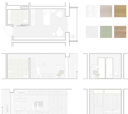
INTERIÉR | M 1:50
