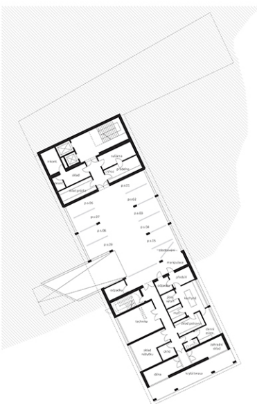
půdorys 1.pp. _ m1:200
