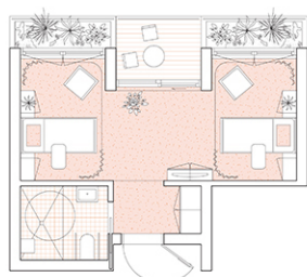
dvojložkový pokoj H _ m1:50
