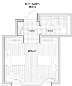
DETAIL DVOULŮŽKOVÉHO POKOJE 1:50
