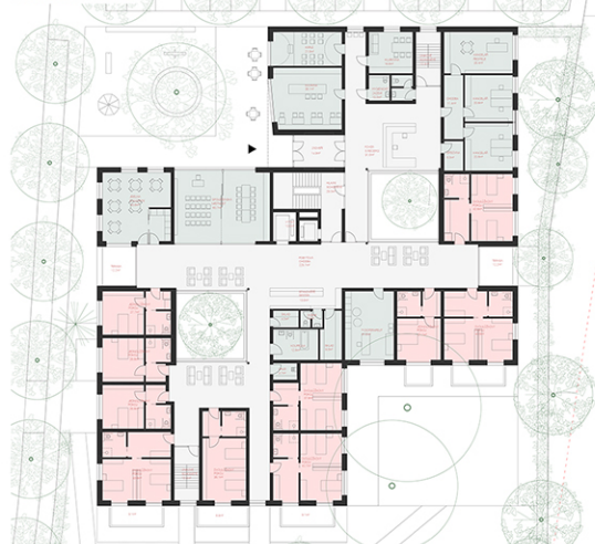
PŮDORYS 1.NP | 1:200
