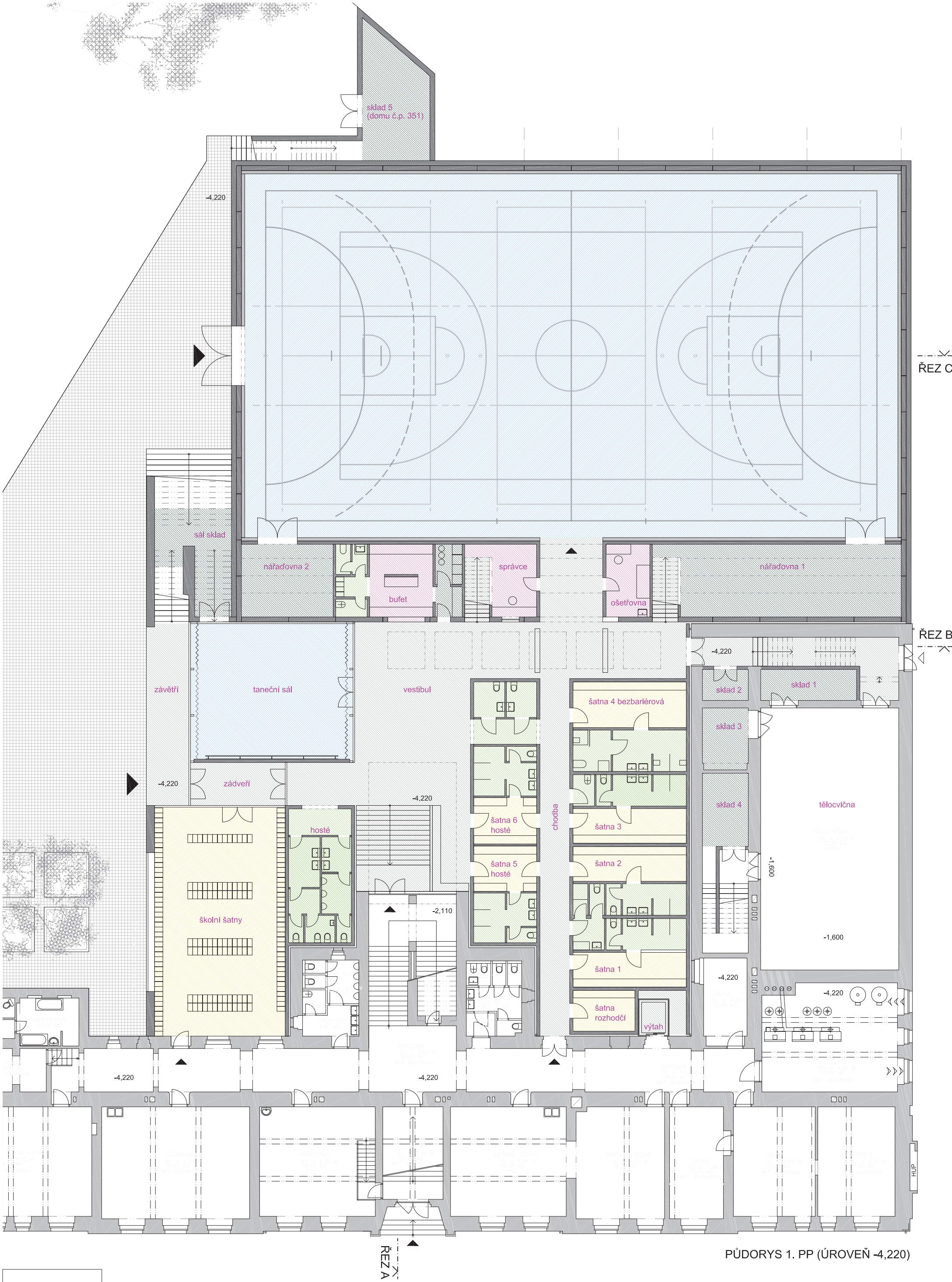
TĚLOCVIČNA U ZŠ VÁCLAVA HEJNY V ČERVENÉM KOSTELCI
